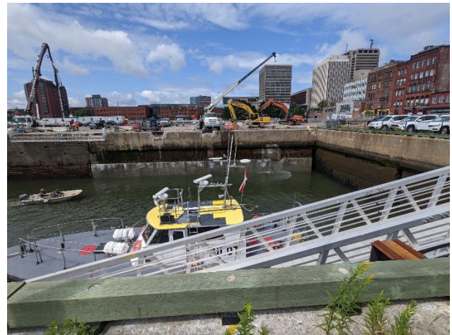
Remplacement d'une partie de la digue à Saint John (N.-B.)
